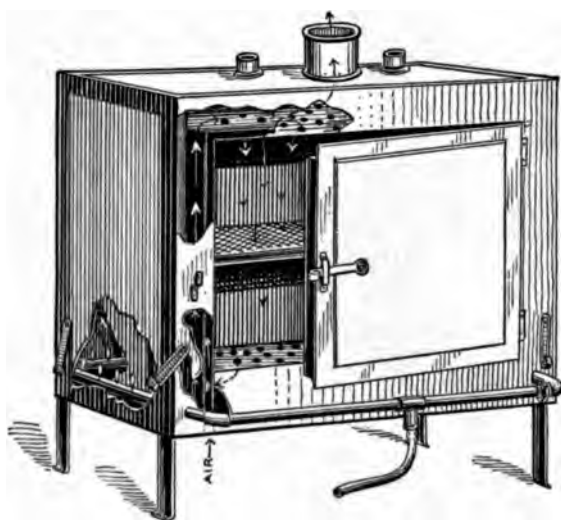
Fig. 2.—Lautenschläger hot-air sterilizer.
